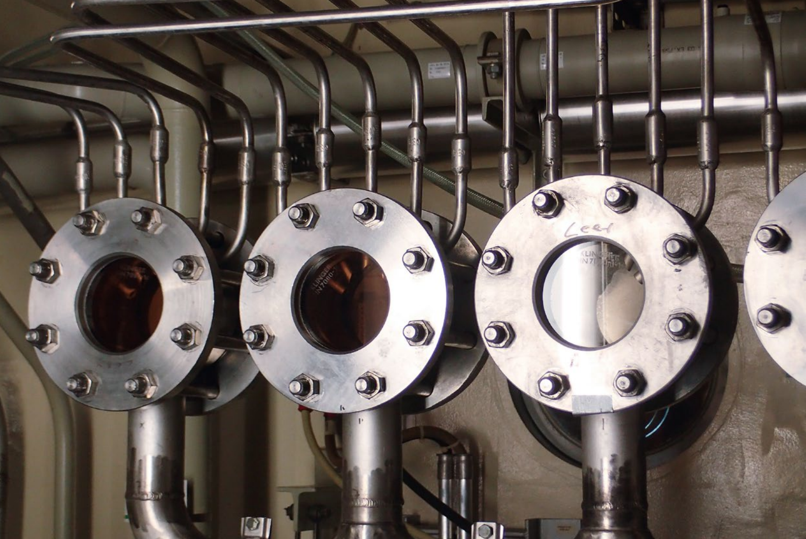
Circuits de mesure dans le bâtiment du réacteur de la centrale nucléaire de Gösgen (photo IFSN)
