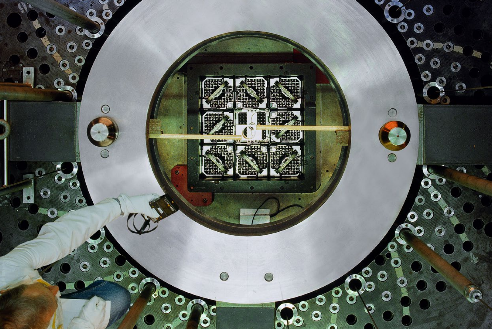
Centre du réacteur de recherche PROTEUS au PSI (entre-temps en désaffectation) (photo PSI)
